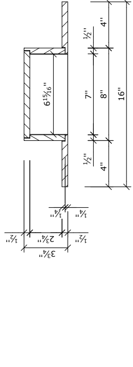
section A-A ( 1 : 5 )
