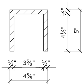
section A-A ( 1 : 5 )
