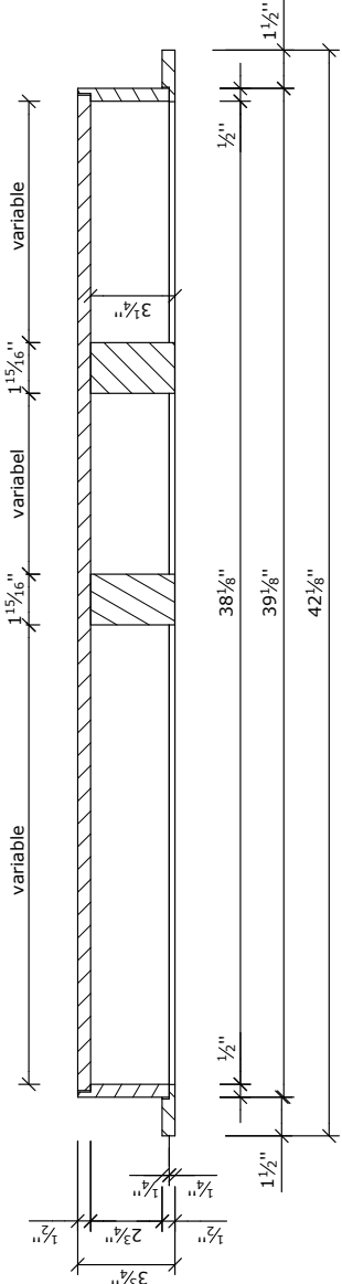
section B-B ( 1 : 5 )
