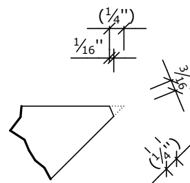
detail A ( 1 : 2 )
